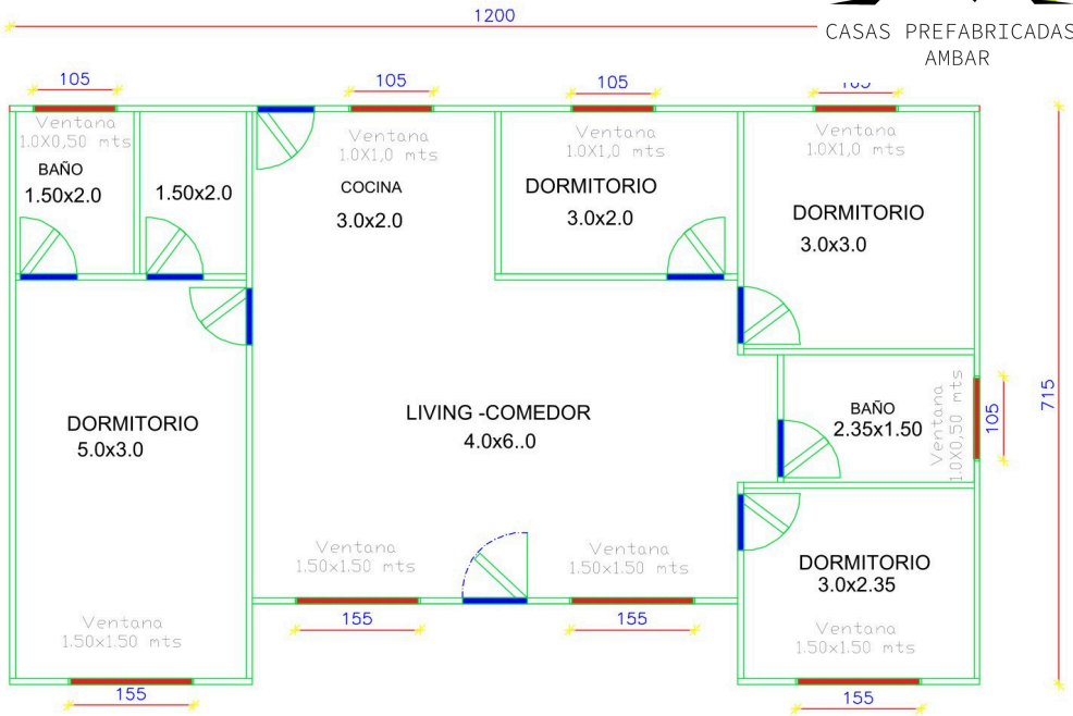
CASA 84 MTS 2 6 AGUAS MAXIMO
